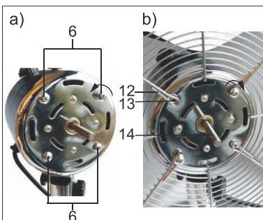
Fig.126: Τοποθέτηση πίσω προστατευτικό πλέγματος
