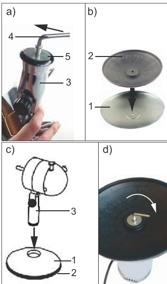
Fig.125: Συναρμολόγηση βάσης
