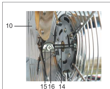
Fig.105: Montáž rotoru
