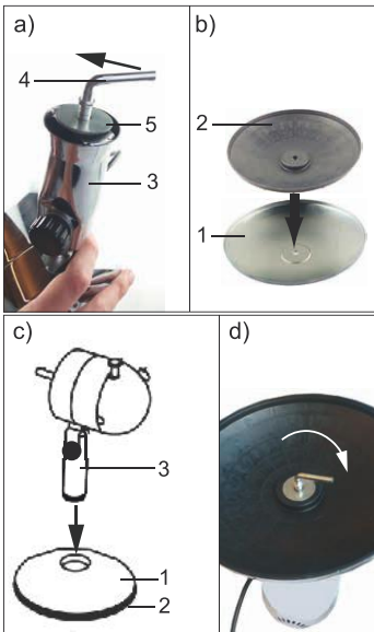
Fig.71: Montaż podstawy
