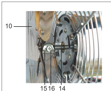
Fig.127: Συναρμολόγηση ρότορα
